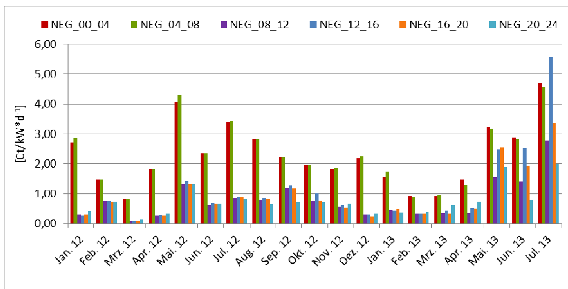
Abb. 3: Durchschnittliche Leistungspreise für negative MRL in den einzelnen Zeitscheiben
