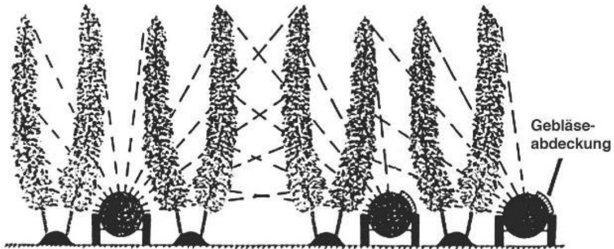
Abb.: Verbesserte Randbehandlung mit TurboDrop-Injektordüsen, zwei einseitigen Spritzfahrten und Abdeckung der äußeren Gebläseaustrittsöffnung
