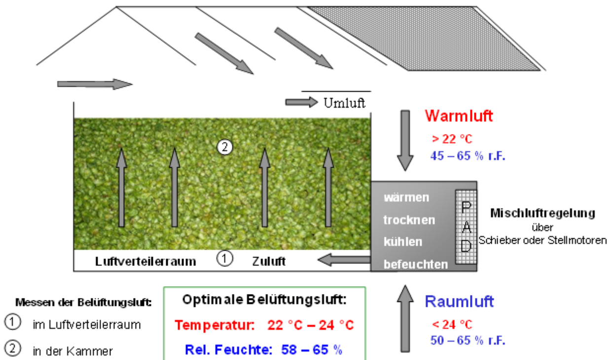
Abb.: Schema der Nachbehandlung von Hopfen in Konditionierungskammern
