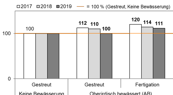
Abb.: Effekte auf den Ertrag (Sorte Perle, Bodenart 03 und 04, Zeitraum 2017 bis 2019)
