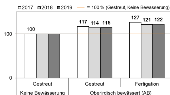
Abb.: Effekte auf den Alphasäuregehalt (Sorte Perle, Bodenart 03 und 04, Zeitraum 2017 bis 2019)
