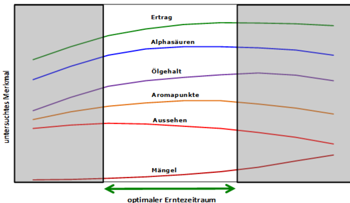
Abb.: Schematischer Verlauf der Qualitätsparameter während der Abreife
