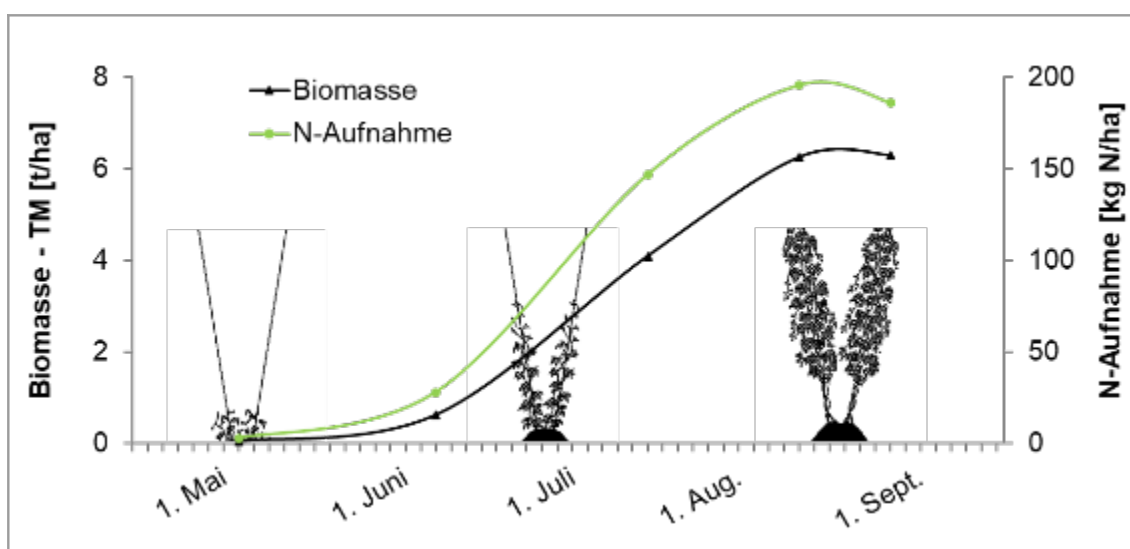
Abb.: Biomasseentwicklung und Stickstoffaufnahme im Vegetationsverlauf von Hopfen
