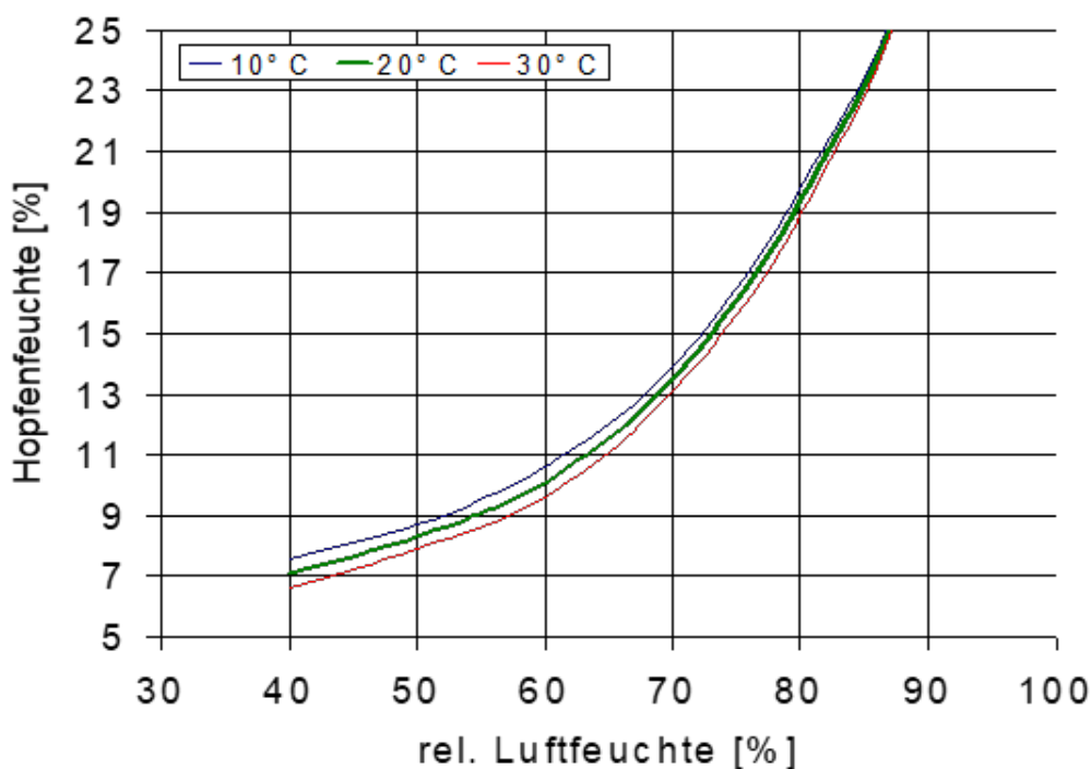
Abb.: Sorptionsisothermen von Hopfen
