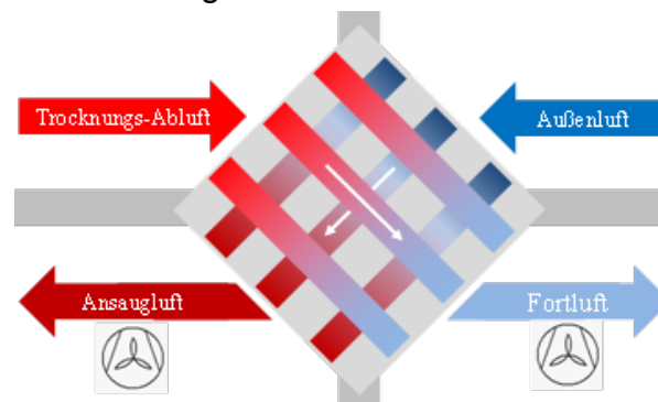
Abb.: Prinzip eines Kreuzstrom-Wärmetauschers
