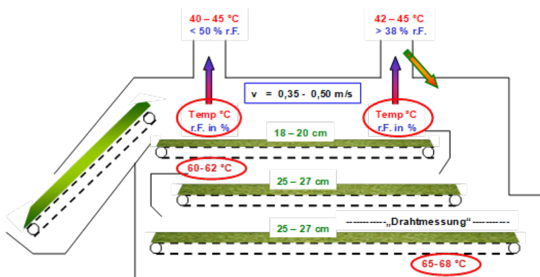
Abb.: Messpunkte und mögliche Grundeinstellungen des Bandtrockners
