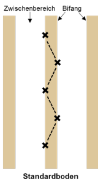
Abb.: Schema der Probenahme
