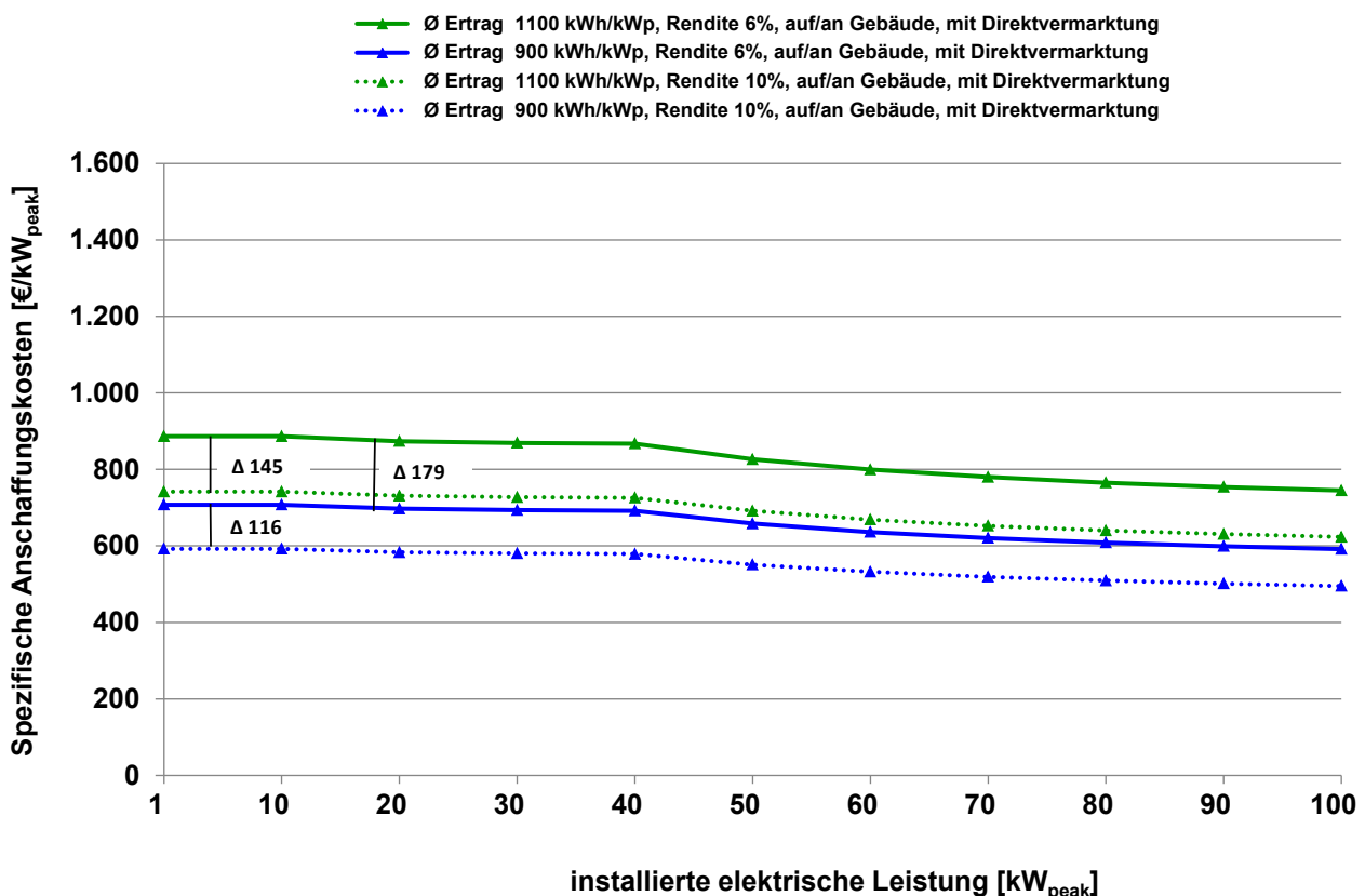
Abbildung 1: „Höchstens tragbare“ Anschaffungskosten einer PV-Dachanlage bis 100 kW p im September 2020
