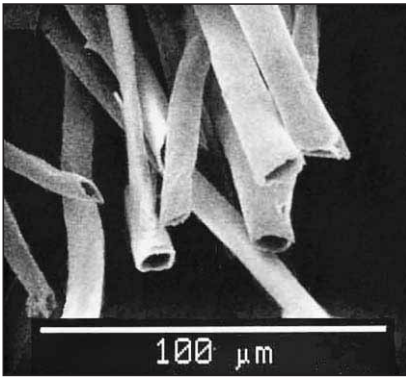
Abb. 8: Mikroskopische Querschnitts- aufnahme der Pappelflaum- Fasern (Foto: PAP(P)ILLON GmbH)
