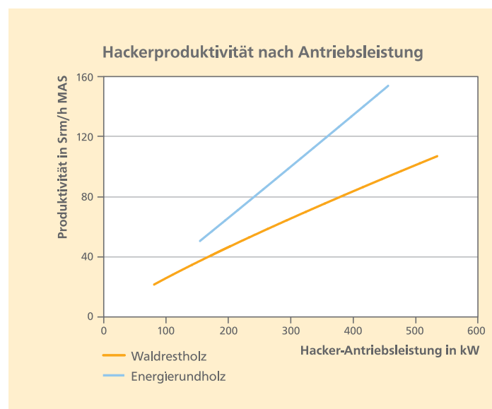
Abbildung 1: Produktivität des Hackers in Schüttraummeter pro Maschinenarbeitsstunde in Abhängigkeit von Ausgangsmaterial und Antriebsleistung
